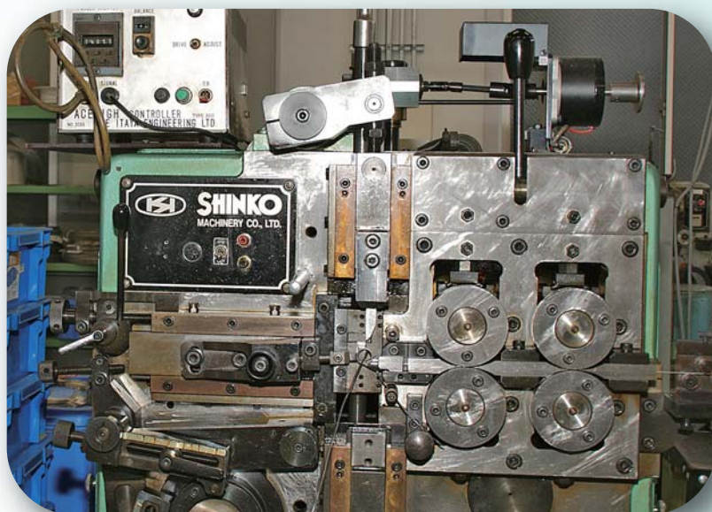
コイリングマシン主要部
